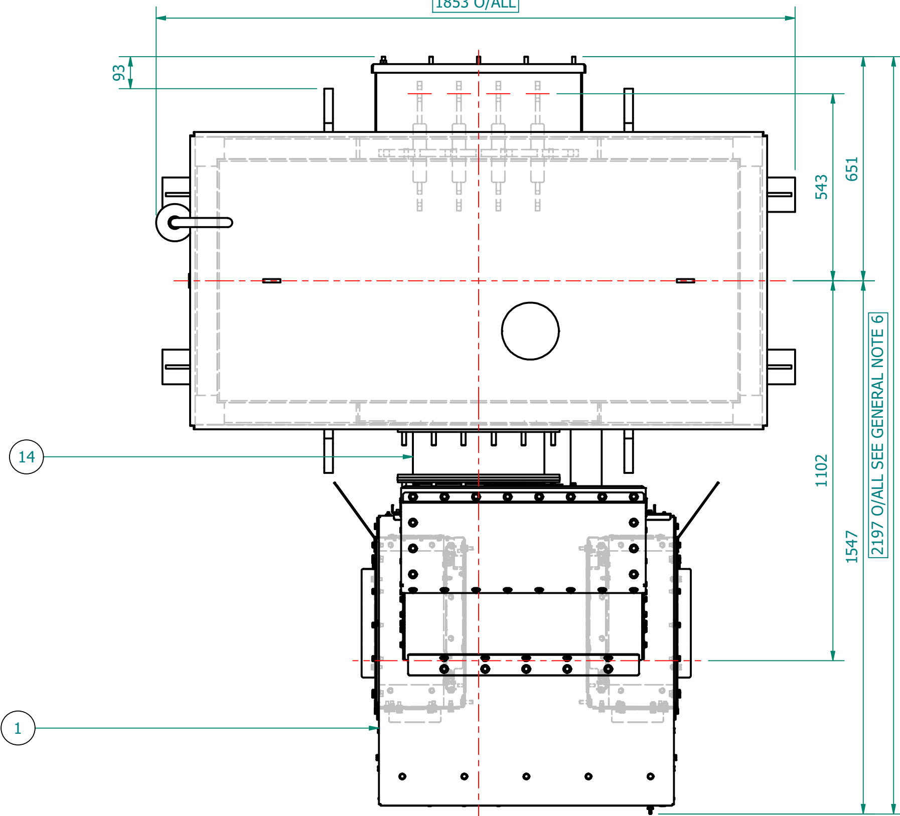
PLAN VIEW 1853 O/ALL
